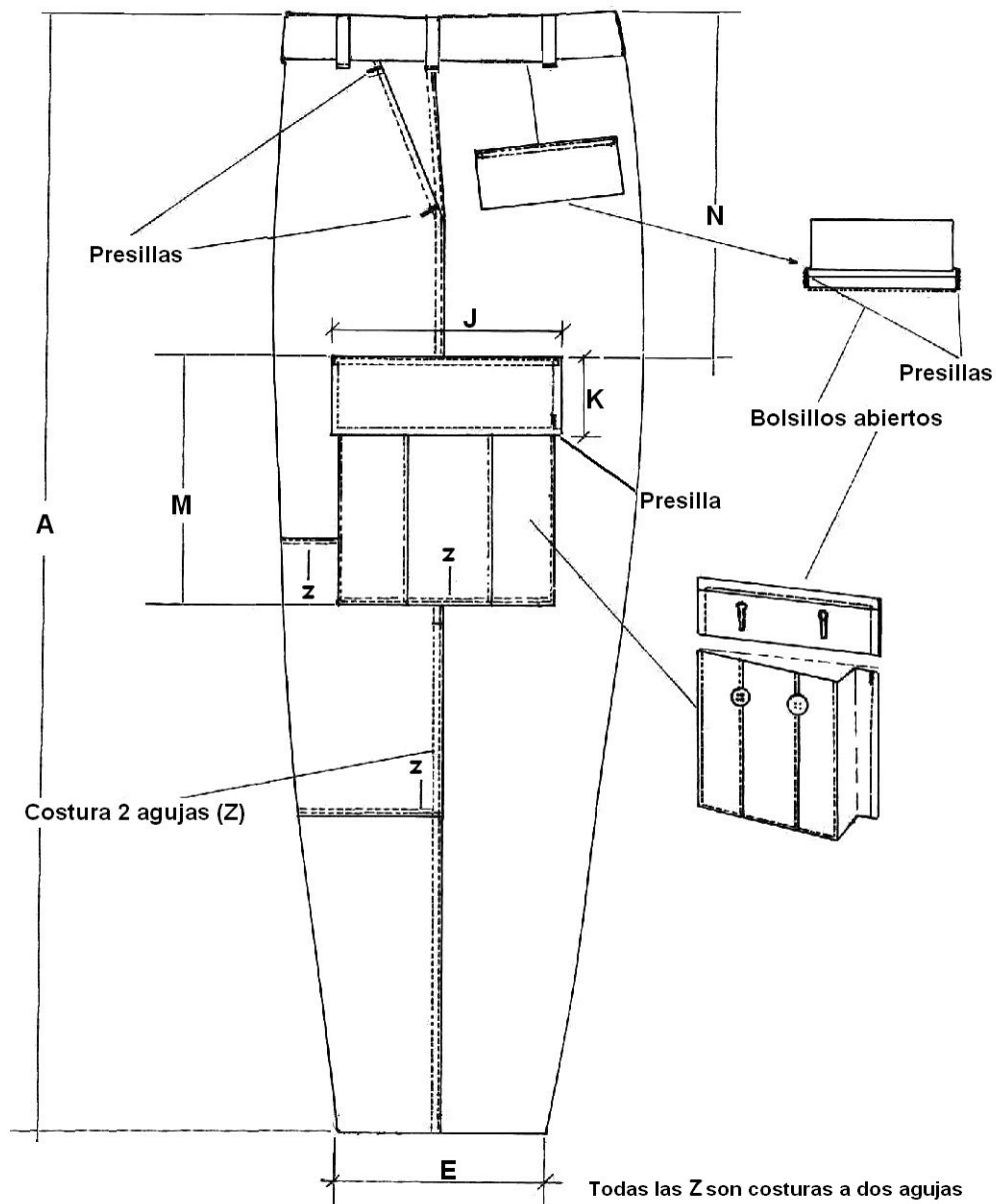
Figura 5. Pantalón vista lateral izquierda
