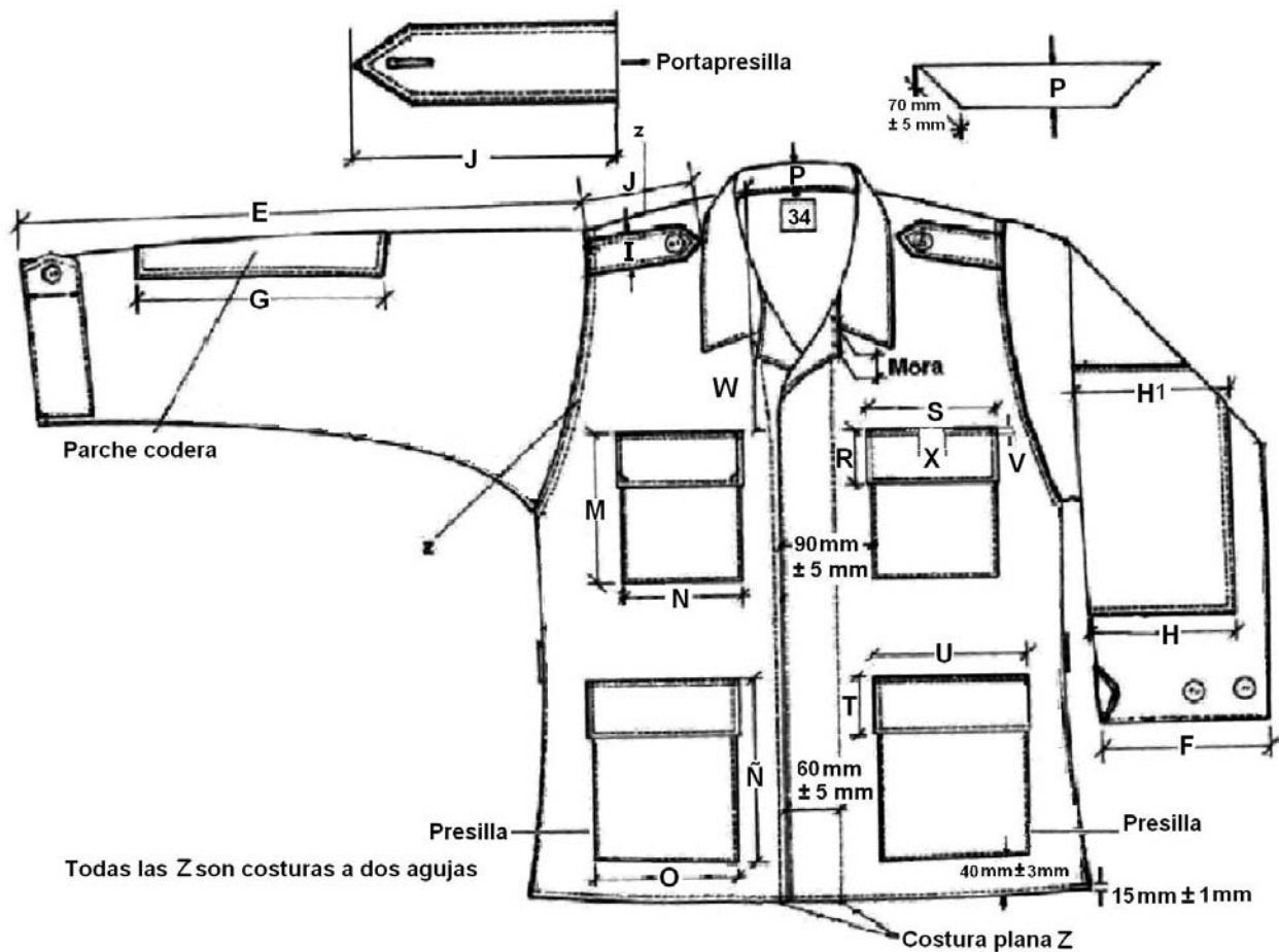
Figura 1. Frente de la camisa
