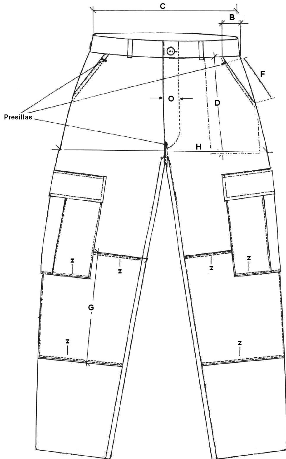
Figura 3. Pantalón vista frontal
