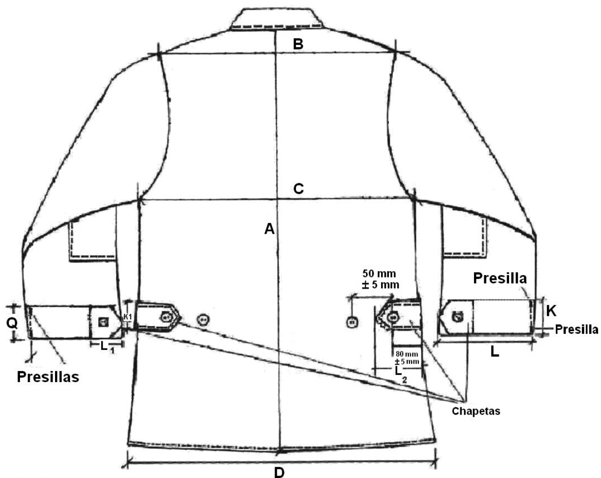
Figura 2. Espaldar de la camisa
